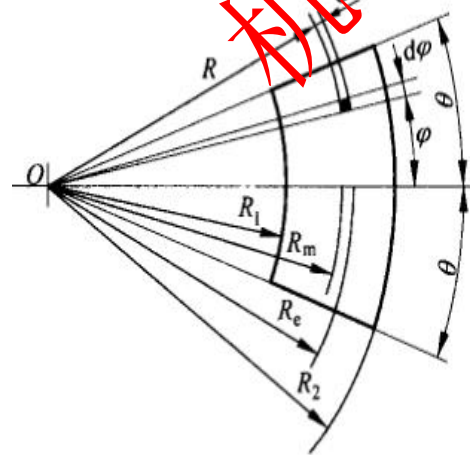
图 5-2 制动力矩计算简图 2
