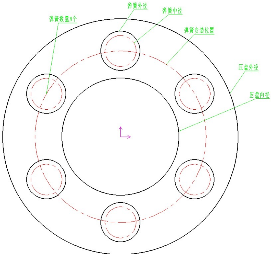
图 4-1 弹簧外径估算用简图
