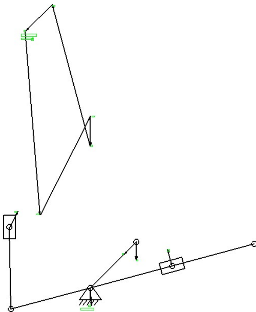
图 3-5 杆组3受力简图
