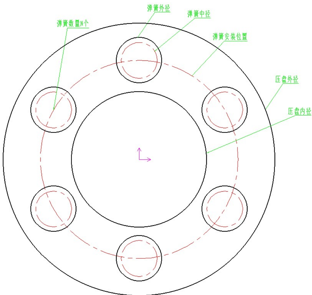
图 4-1 弹簧外径估算用简图
