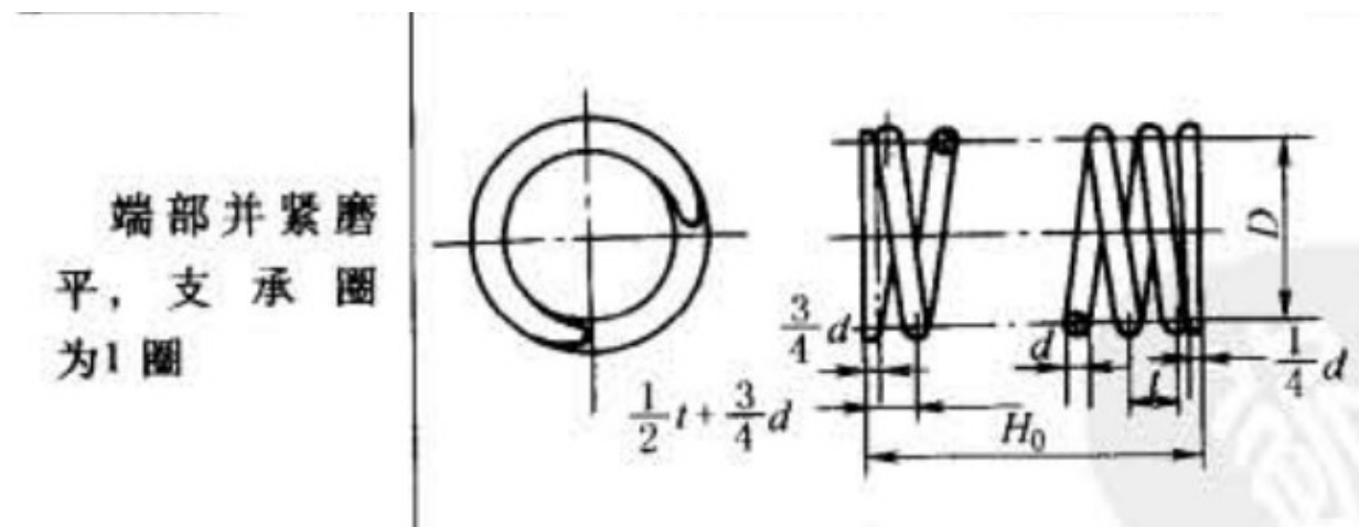
图 4-1 弹簧结构简图
